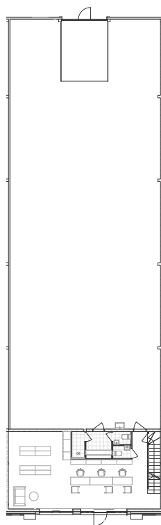
1.KORRUS
